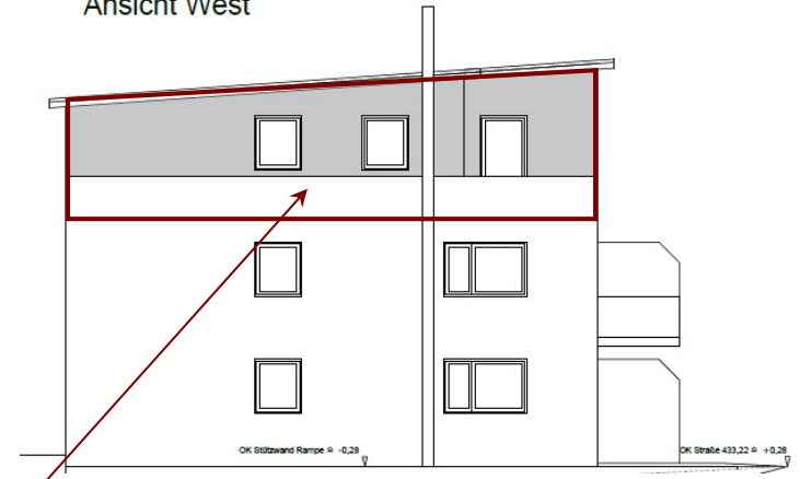
Ansicht West
